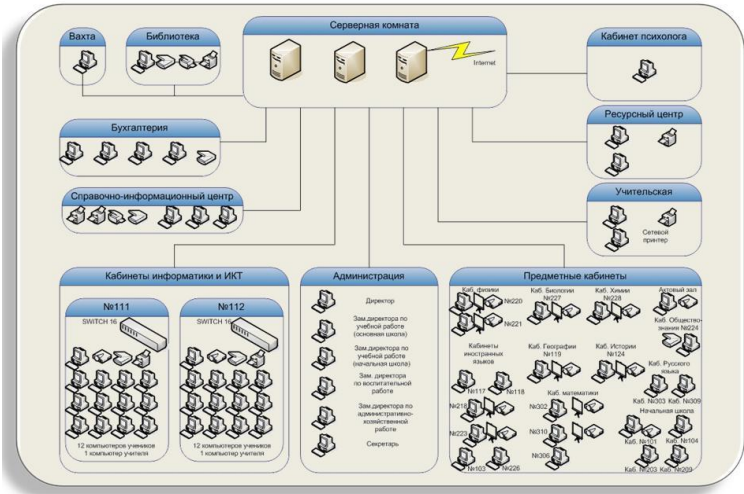
Схема локальной сети ОУ
